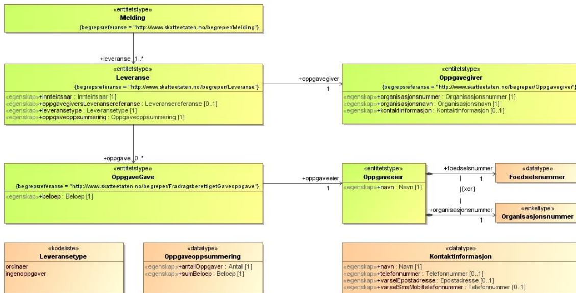
Figur 2 – Dokumentstruktur (UML)
