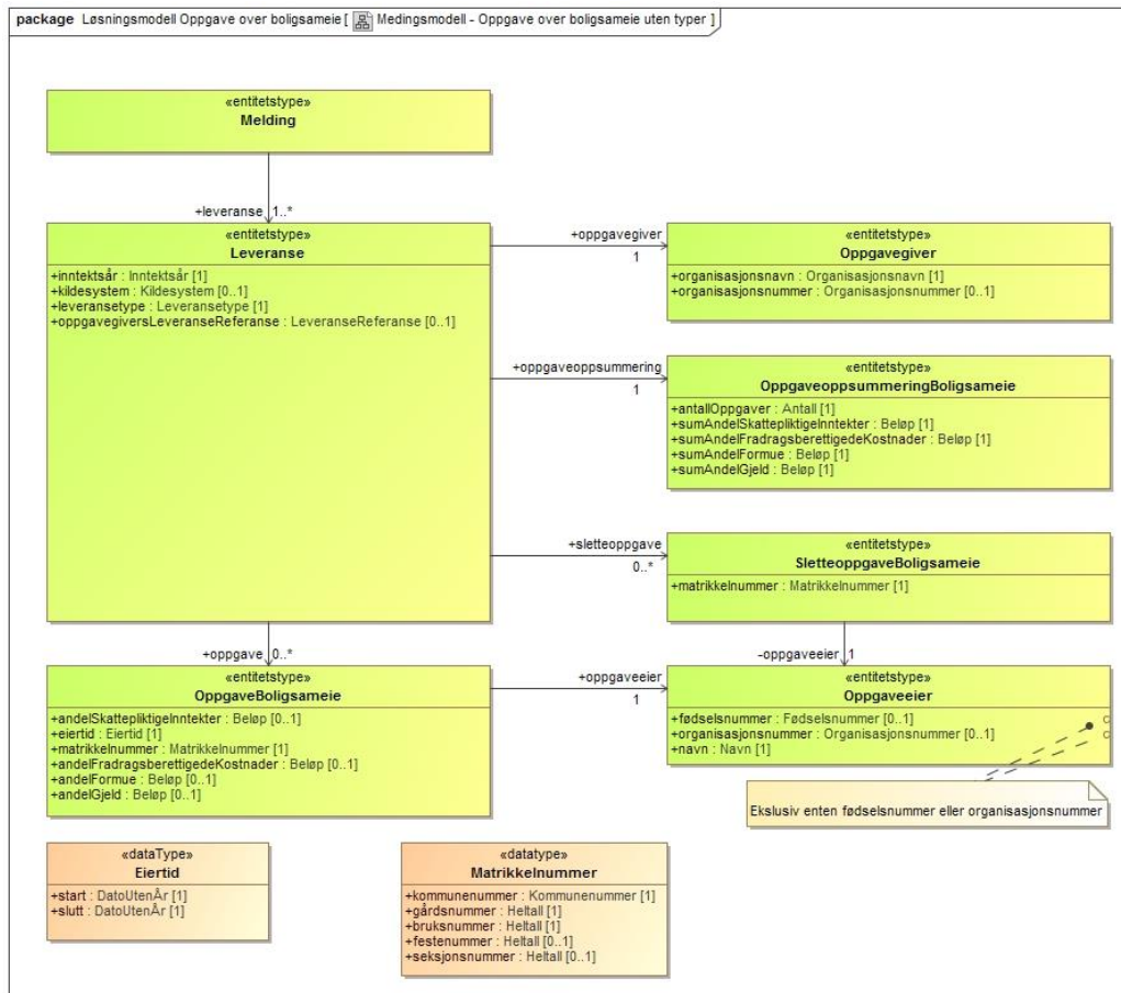
Figur 2 – Dokumentstruktur (UML)
