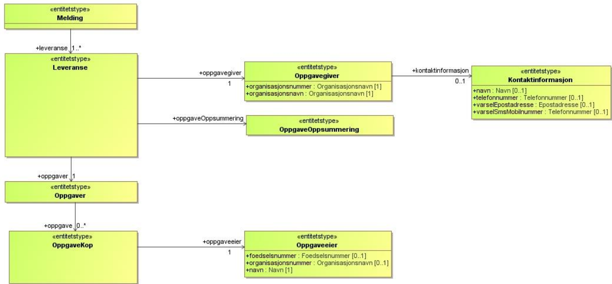
Figur 2 – Dokumentstruktur (UML)
